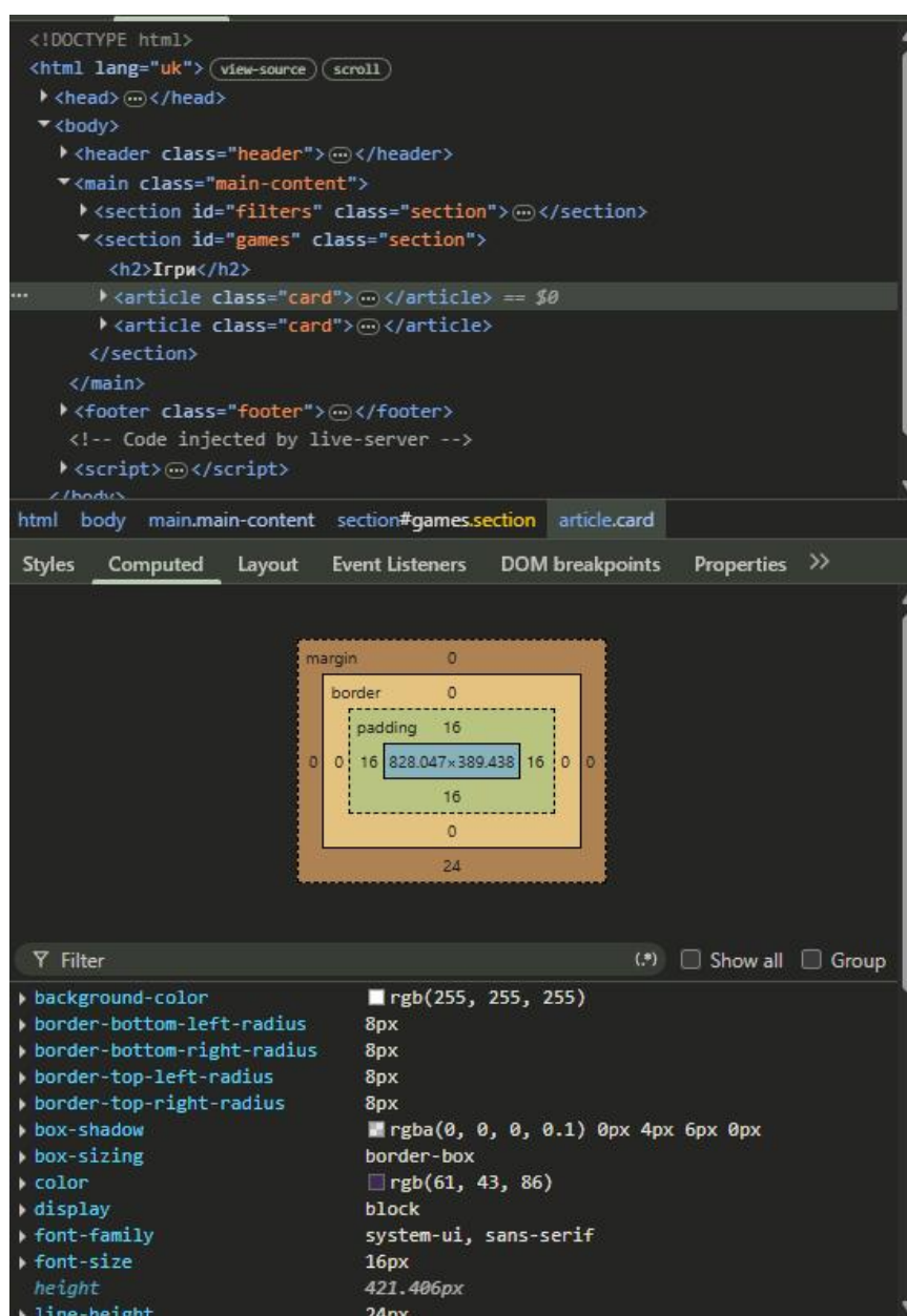
Рис. 7 — Діаграма box model для елемента article у DevTools
